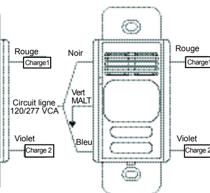
Capteur pour deux circuits (câblé pour un circuit)
