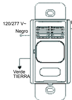
Circuito simple
