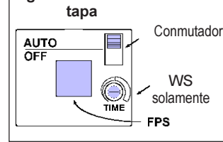
Fig. 2 - Vistas detrás de la tapa
