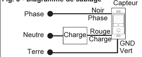
Fig. 3 - Diagramme de câblage
