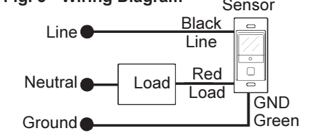
Fig. 3 - Wiring Diagram
