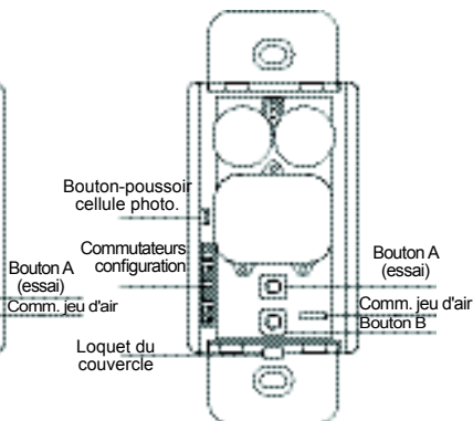
Capteur à deux boutons
