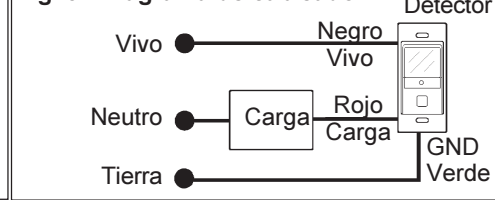
Fig. 3 - Diagrama de cableado
