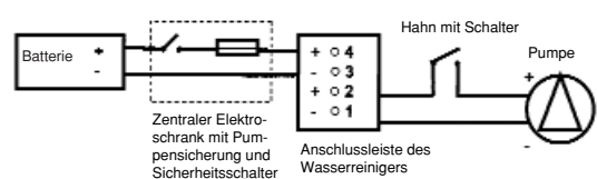
Schalergesteuerte Pumpe mit Wasserreiniger
