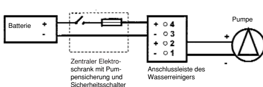
Druckgesteuerte Pumpe mit Wasserreiniger
