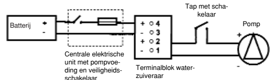
Schakelaargeregelde pomp met waterzuiveraar
