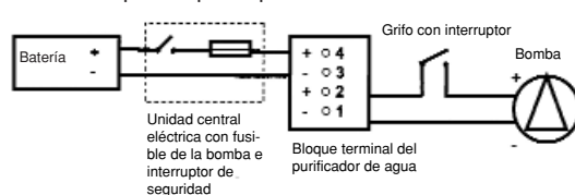
Bomba con control por interruptor con purificador
