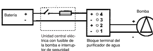
Bomba con control por presión con purificador
