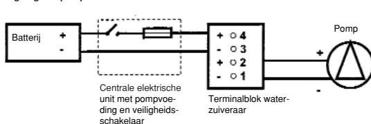
Drukgeregelde pomp met waterzuiveraar
