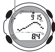
気圧差グラフィック(+5hPa)
