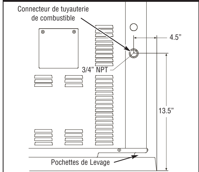
Figure 30 — Emplacement du Combustible et des Éléments
