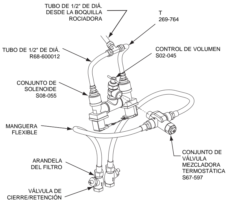
CONJUNTO DE VÁLVULA S50-369
