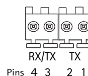
RS-485/422
